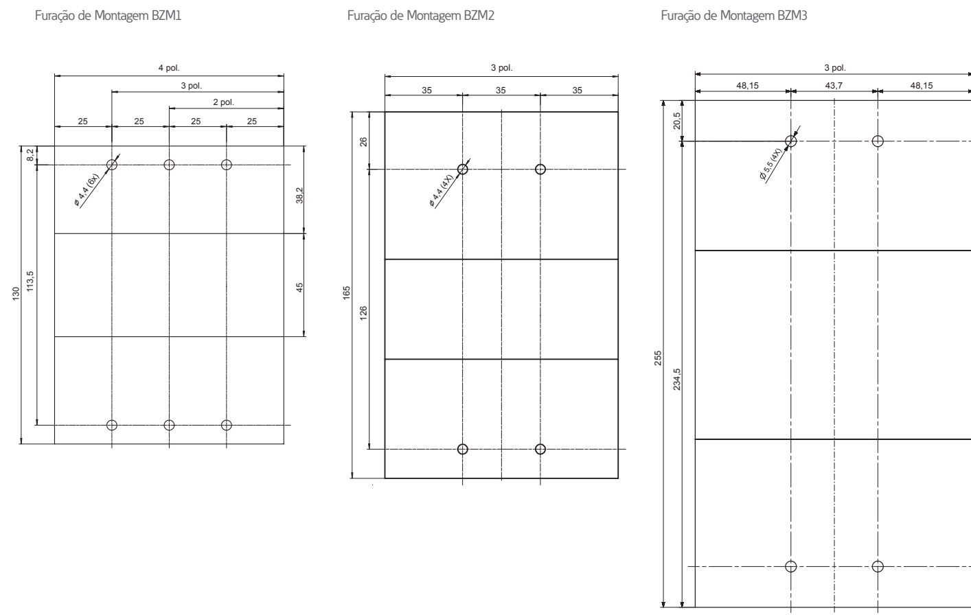
Furação de Montagem BZM1, BZM2 e BZM3
