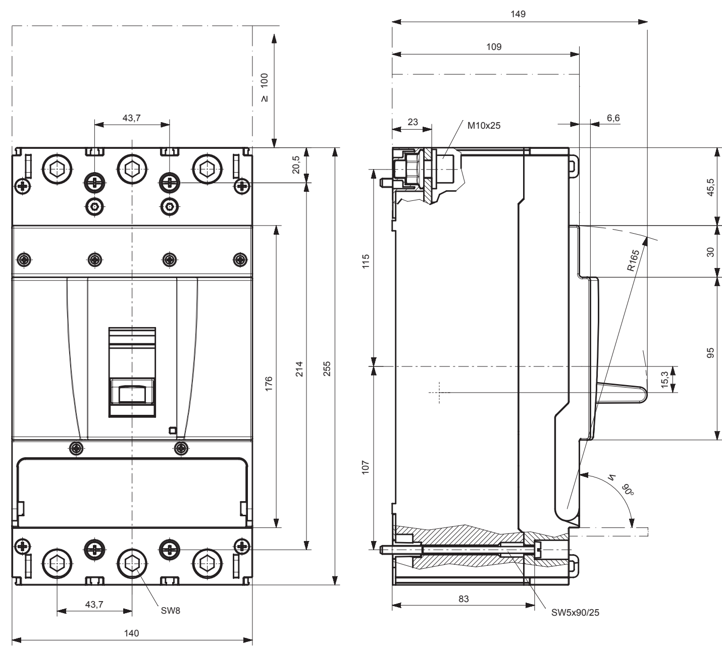
Disjuntor BZM3 Posição de Montagem BZM1 / BZM2 / BZM3
