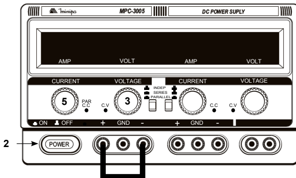
Figura 4 – Ajuste da Corrente Limite
