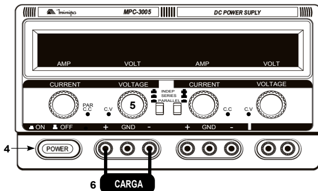
Figura 6 - Conexão das Fontes MPC-3003 e MPC-3005.
