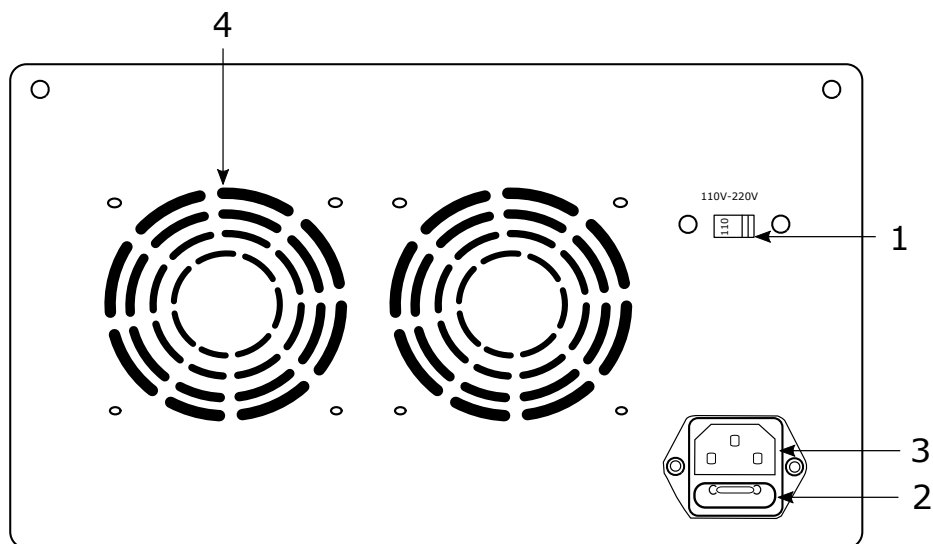
Figura 2 – Painel Traseiro Fontes MPC-3003 e MPC-3005
