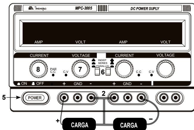
Figura 9 - Conexão Simétrica das Fontes MPC-3003 e MPC-3005.
