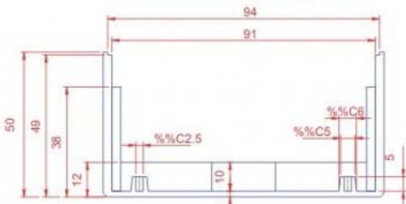
CORTE-AA
