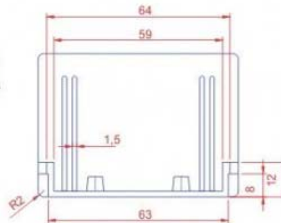
CORTE-BB
