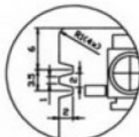
DETALHE-A ESC: 31
