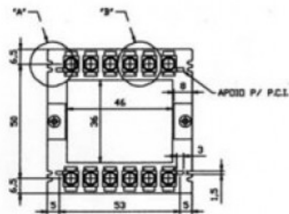
DETALHE-B ESC: 31
