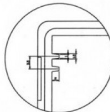
DETALHE - 1/4 ESC. 41
