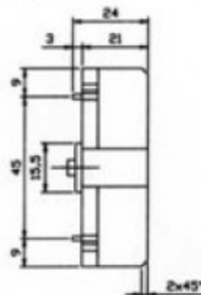
DETALHE-A ESC: 31
