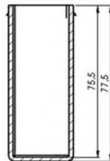
SEÇÃO A-A
