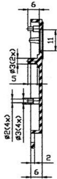
CORTE-AA
