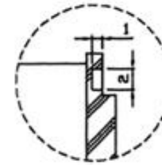
DETALHE - 'B' ESC: 3:1
