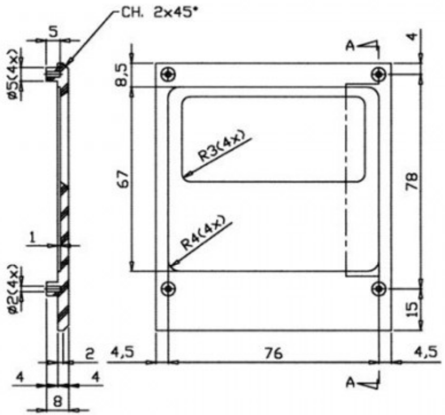
CORTE-AA
