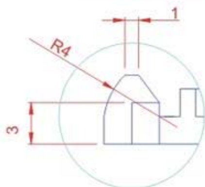
DETALHE - "A" ESC.: 3:1
