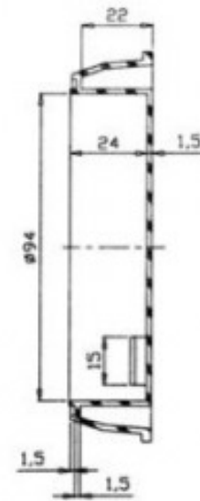
CORTE-BB
