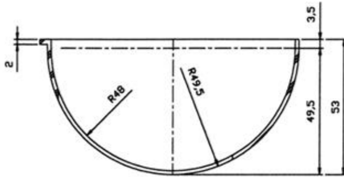
CORTE-AA
