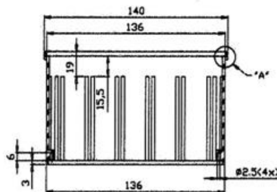
CORTE-AA
