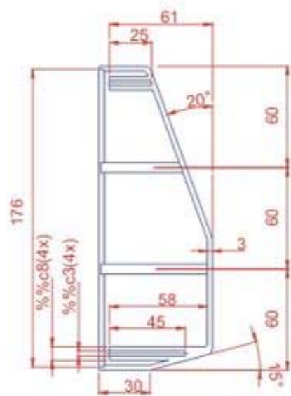
CORTE-BB
