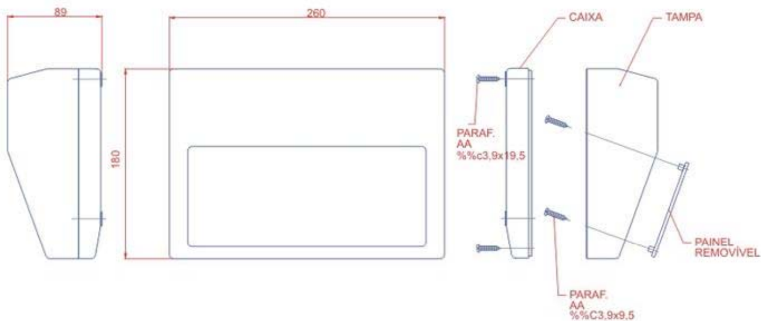
PERSPECITVA S:E
