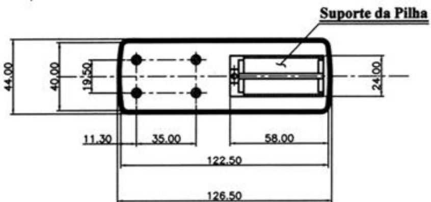
CORPO
