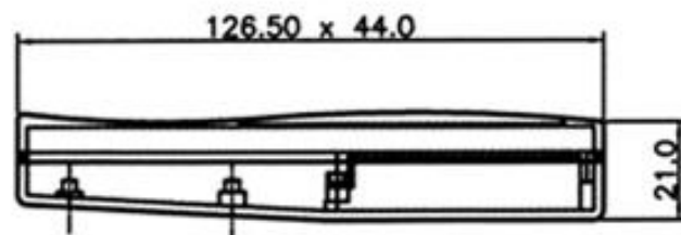
CAIXA MONTADA
