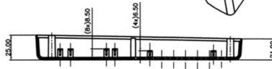
CORTE " B-B "
