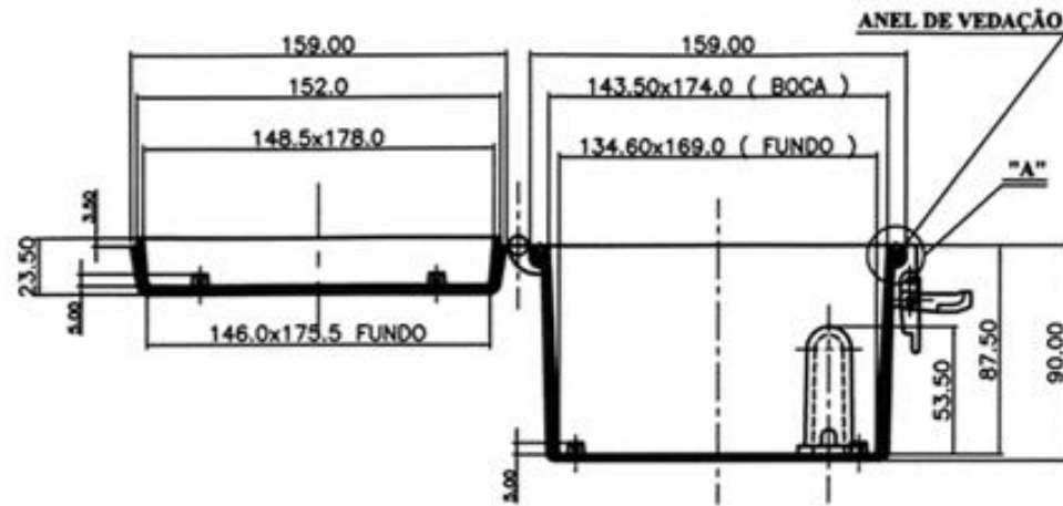
SECCÃO "A"
