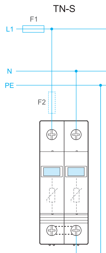
(2x) 7P.21.8.275.1020 + (1x) 07P.22
