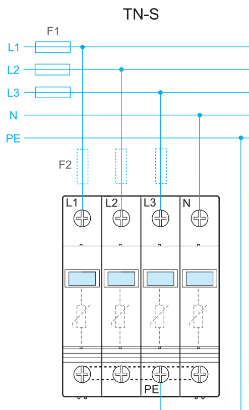
(4x) 7P.21.8.275.1020 + (1x) 07P.24
