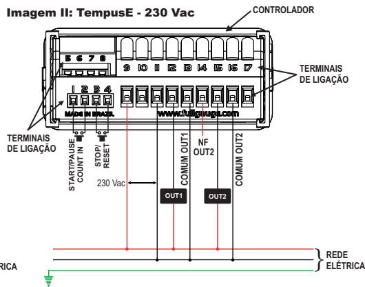
Imagem II: TempusE - 230 Vac
