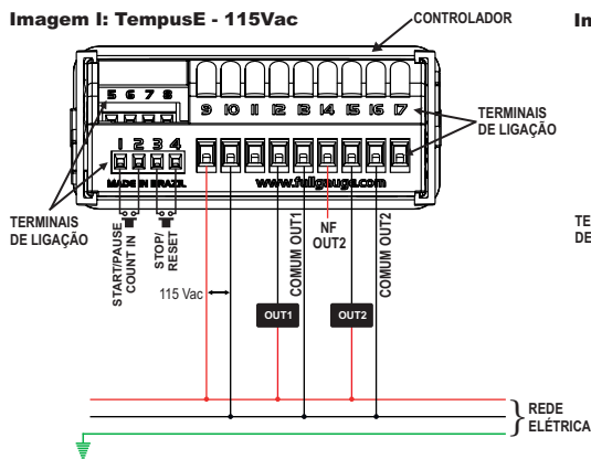
Imagem I: TempusE - 115Vac
