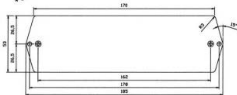
DETALHE "A" ESC. 3:1
