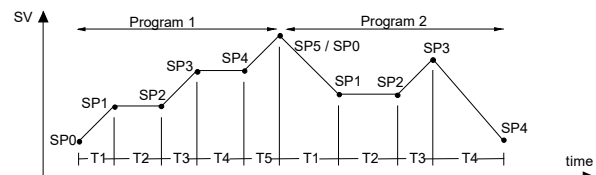
Fig. 11 - Exemplo de programa 1 e 2 interligados
