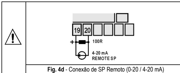
Fig. 4d - Conexão de SP Remoto (0-20 / 4-20 mA)
