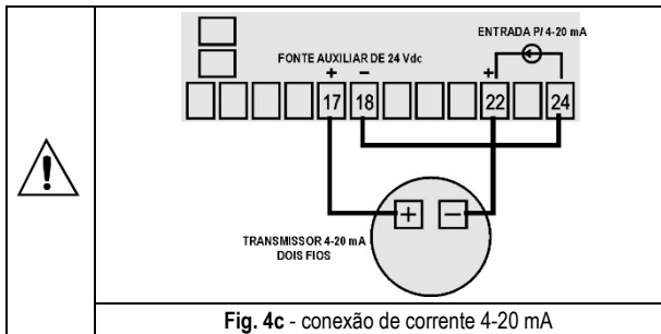
Fig. 4c - conexão de corrente 4-20 mA
