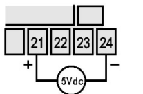
Fig. 4b - Conexão de tensão 5 Vcc
