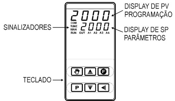
Fig. 8 - Identificação das partes do painel frontal
