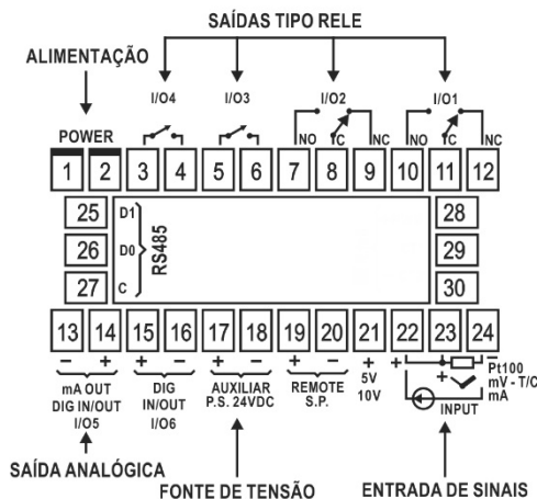
Fig. 1 - Conexões do painel traseiro
