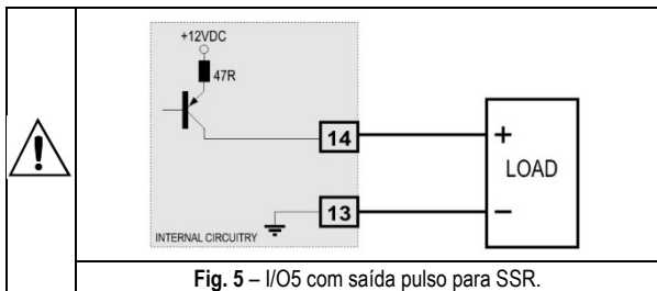
Fig. 5 - I/O5 com saída pulso para SSR.
