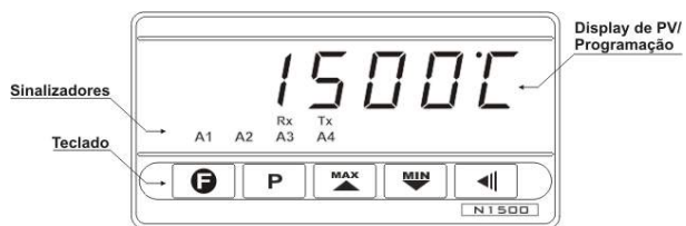
Fig. 10 - Identificação das partes do painel frontal
