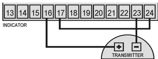
Fig. 9 – Transmissor a 2 fios utilizando a fonte de 24 Vcc do indicador
