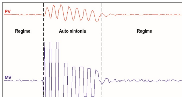
Figura 11 - Exemplo de uma auto sintonia
