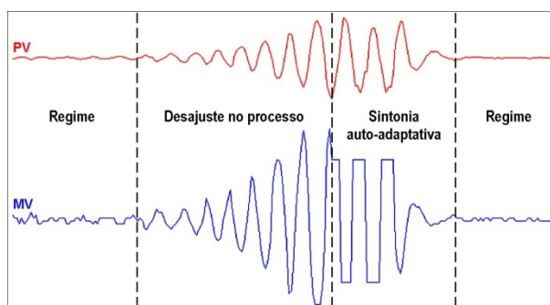
Figura 12 - Exemplo de uma sintonia auto-adaptativa
