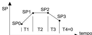
Figura 9 - Exemplo de programa com poucos segmentos
