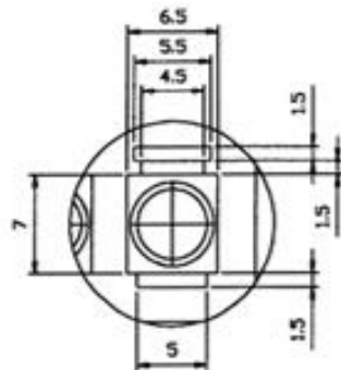
DETALHE - "A" ESC:3/1
