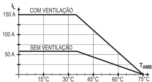
Fig. 3 – Dissipador NDP3 (para 120 mm: R thja = 0,52 / 0,12 °C / W)
