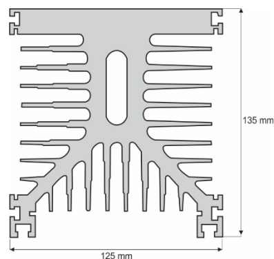
Fig. 6 – Dissipador NDP3 (para 120 mm: R thja = 0,52 °C / W)
