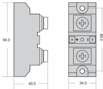
Fig. 7 – Dimensões do SSR
