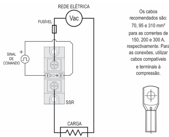
Fig. 2 – Conexões Elétricas – Sinal de comando e Carga
